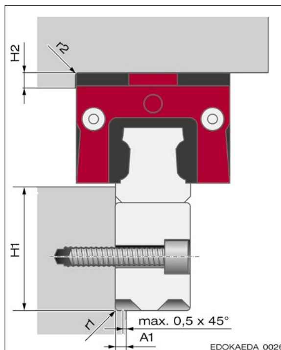
Gestaltung der Anschlusskonstruktion
