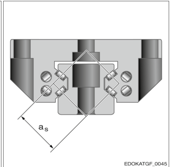
O-Geometrie mit Stützabstand a_s
