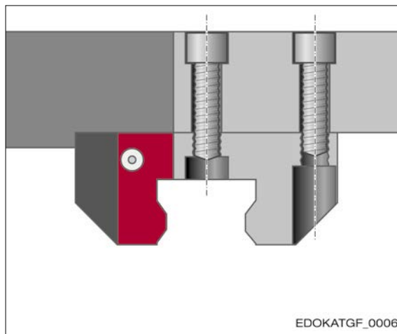
Befestigung unter Verwendung der Gewindebohrung
