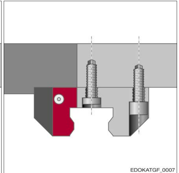
Verwendung der Führungswagenbohrung als Durchgangsbohrung
