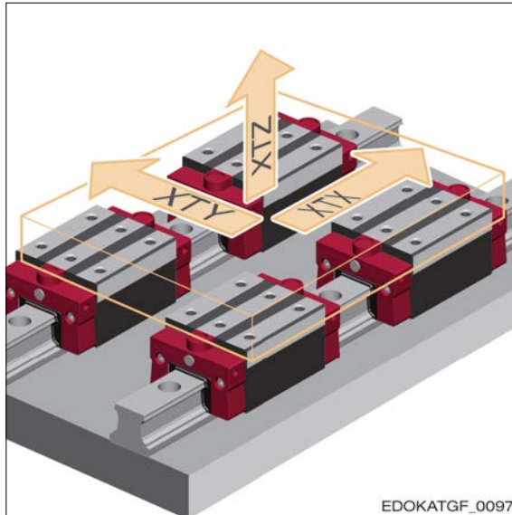
Translationsbewegung von 4 verbundenen Führungswagen
