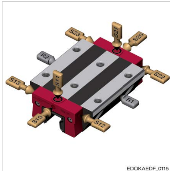
Schmieranschlüsse des Führungswagens für Standardschmierung
