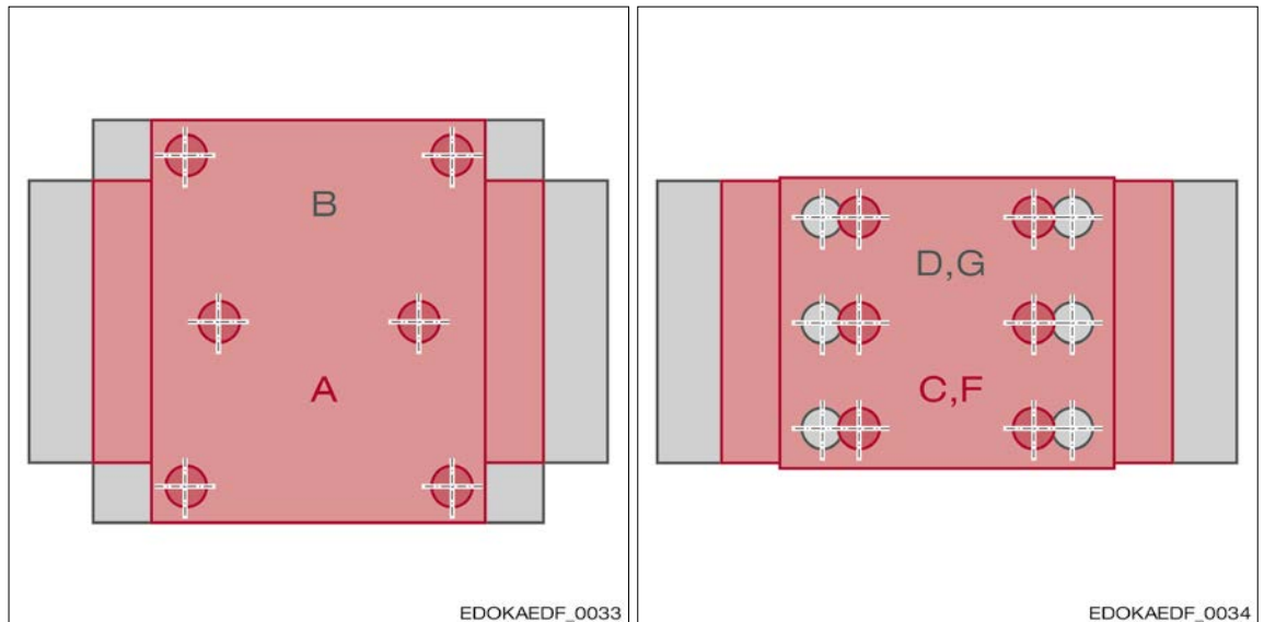
Anschraubbohrbilder für Führungswagenbauform A und B
