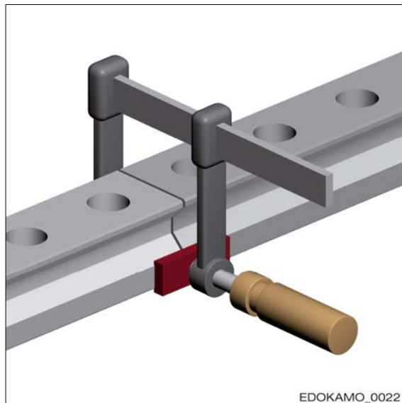
Montage mit Fixierbrücke
