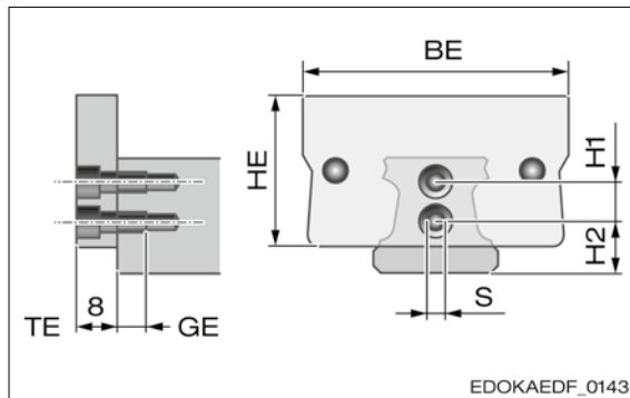
Abmessungen und Stirnbohrungen in der Führungsschiene
