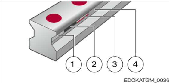
Magnetischer Maßstab
