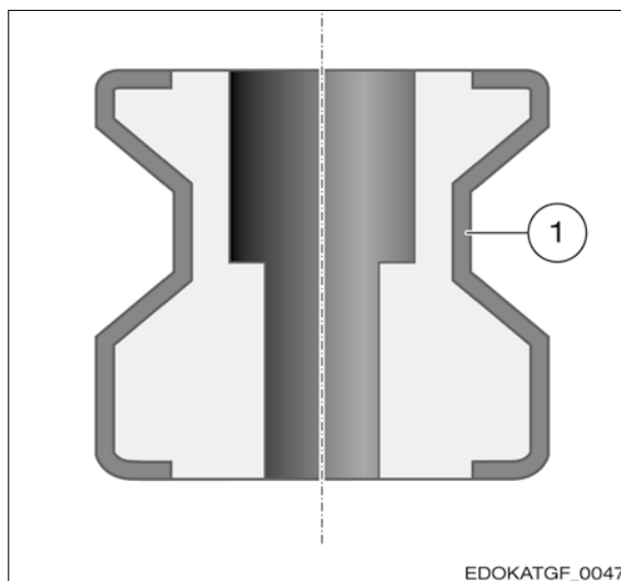
Induktiv gehärtete Führungsschiene mit Härtezone (1) am Beispiel einer MR Führungsschiene
