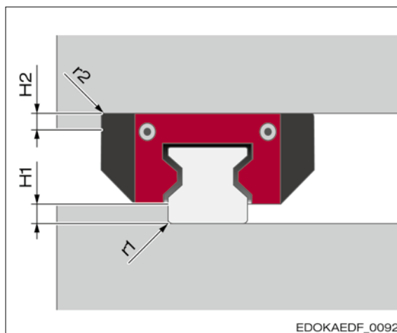
Abmasse der Anschlusskonstruktion
