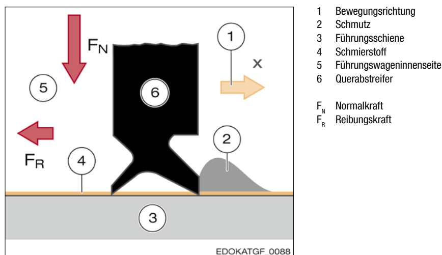
Funktion eines Querabstreifers (im Querschnitt) in der Bewegungsrichtung (gelber Pfeil).
