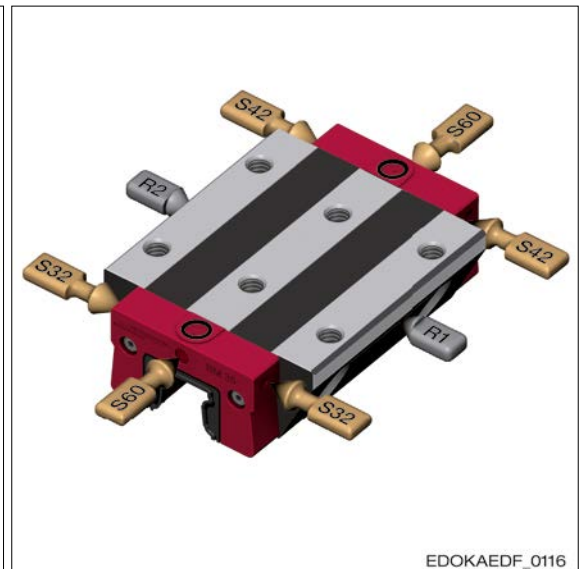
Schmieranschlüsse des Führungswagens für unabhängige Schmierung der Laufbahnen
