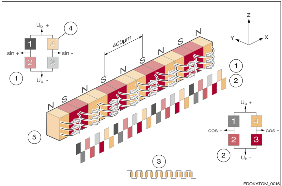
Schematischer Sensoraufbau:
