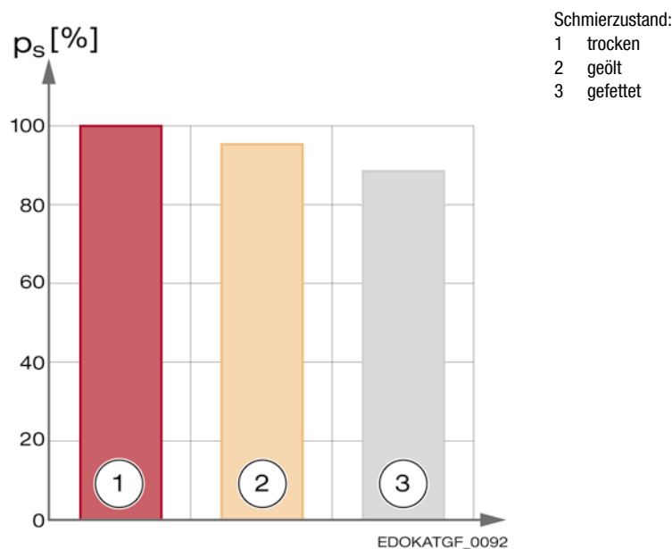
Geräuschentwicklung einer Kugelführung BM 35 in Abhängigkeit von der Schmierung. Der Schmierzustand ist gegen den Schalldruck p_s (%) aufgeführt.
