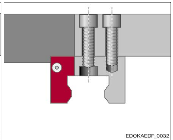
Befestigung unter Verwendung der Gewindebohrung
