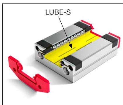
Langzeitschmierung LUBE-S
