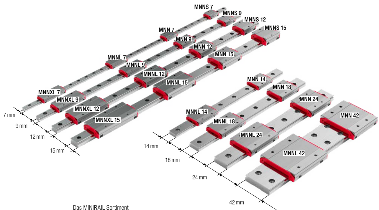
Das MINIRAIL Sortiment
