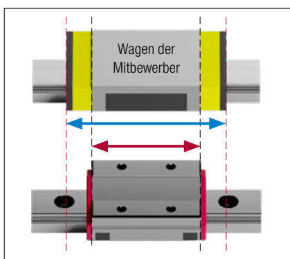
Die Wagenlänge bleibt mit LUBE-S unverändert Folglich werden die Verfahrwege nicht beeinträchtigt
