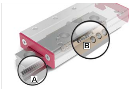
Die robuste Käfigzwangssteuerung von MINISLIDE MSQ
