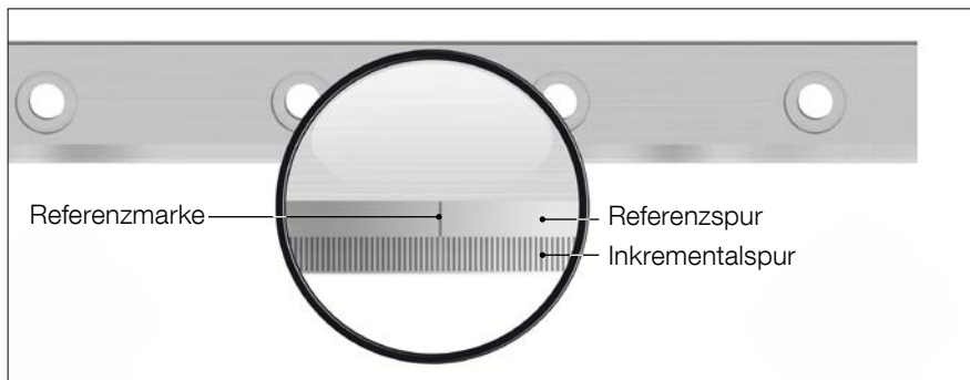
MINISCALE PLUS Schiene mit Massverkörperung
