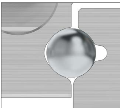
Gotisches Profil der Führungslaufbahnen
