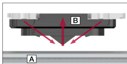
Sensorprinzip
