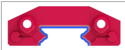
Abstreifer Standard (blaue Kontur = Kontaktfläche)
