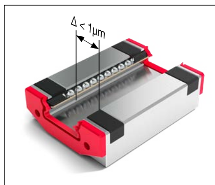
Einheitswagen-System
